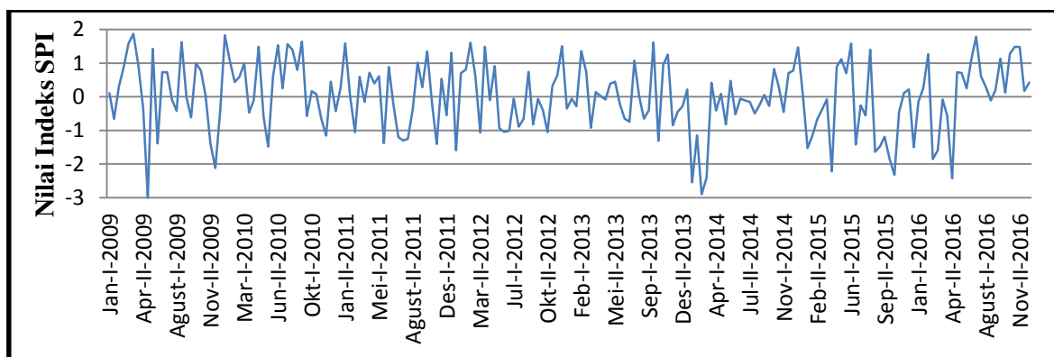
Gambar 1 . Grafik Nilai Indeks Kekeringan SPI Periode 2 minggu BB7
