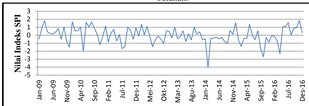
Gambar 2. Grafik Nilai Indeks Kekeringan SPI bulanan BB7
