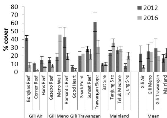
Gambar 7. Histogram rata-rata (± SE) persentase tutupan karang keras pada setiap lokasi penelitian tahun 2012 dan 2016.
