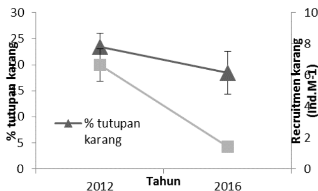
Gambar 6. Rata-rata (± SE) persentase tutupan karang (▲) dan rekrutmen karang (■) di TWP Gili Matra.
