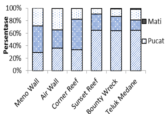
Gambar 4. Histogram komposisi pemutihan karang pada setiap lokasi pengamatan.
