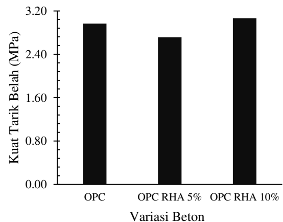
Gambar 6. Hasil Pengujian Kuat Tarik Belah Beton
