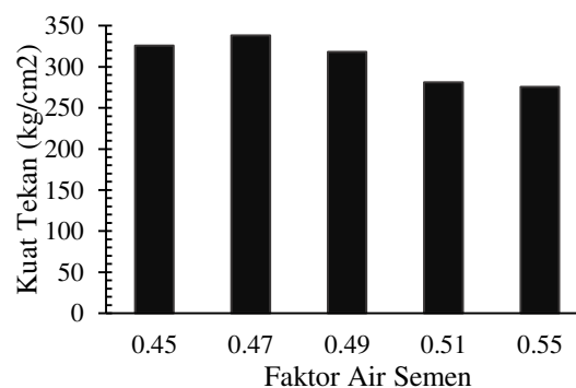
Gambar 3. Grafik hubungan FAS dengan Kuat Tekan Beton Trial Mix
