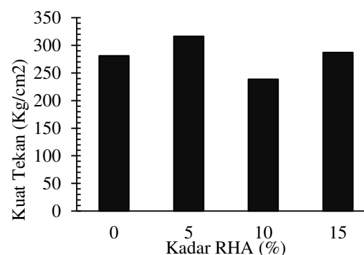
Gambar 4. Grafik hubungan Kadar RHA dengan Kuat Tekan Beton Trial Mix
