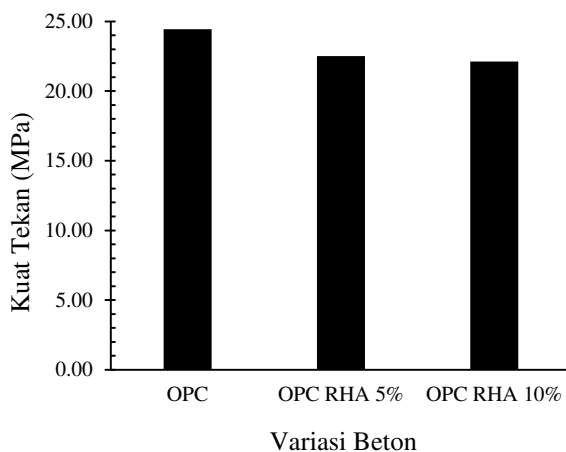
Gambar 5. Hasil Pengujian Kuat Tekan Beton
