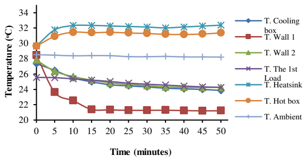
Gambar 9. Pengujian satu beban pendingin
