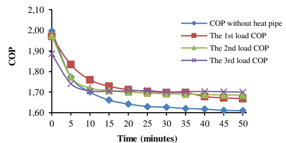
Gambar 12. COP Pengujian pendingin dan pemanas portable tanpa heat pi pe
