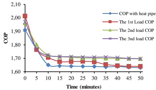
Gambar 13. COP Pengujian pendingin dan pemanas portable dengan heat pipe
