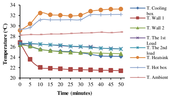
Gambar 10. Pengujian dua beban pendingin
