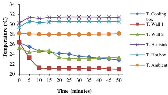
Gambar 8. Pengujian tanpa beban pendingin
