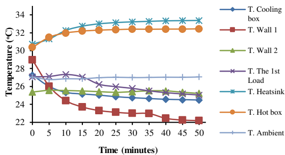
Gambar 5. Pengujian satu beban pendingin
