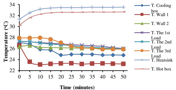
Gambar 7. Pengujian tiga beban pendingin
