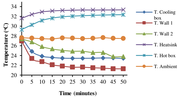
Gambar 4. Pengujian tanpa beban pendingin
