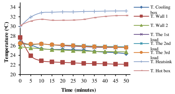
Gambar 11. Pengujian tiga beban pendingin
