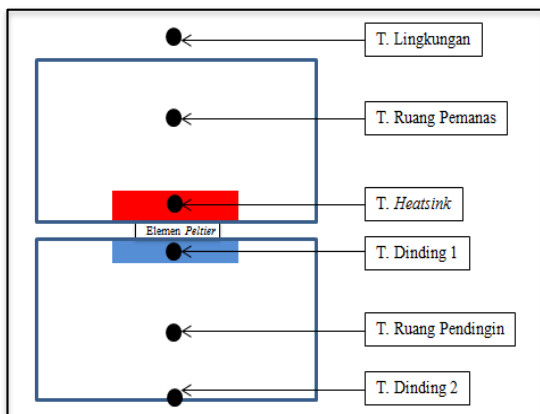
Gambar 2. Metode pengambilan data
