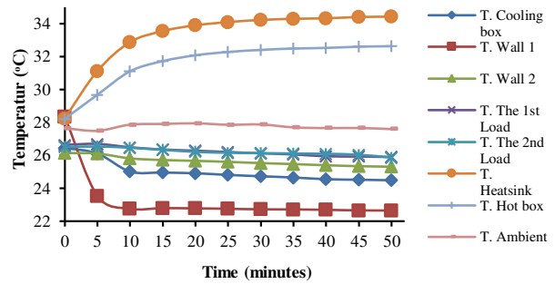
Gambar 6. Pengujian dua beban pendingin
