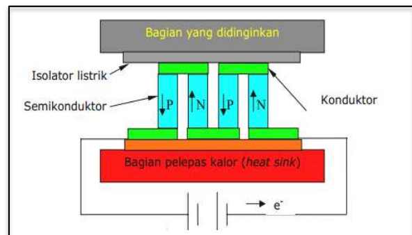
Gambar 1. Skema Aliran Elektron pada Element Peltier Tellurex [4]
