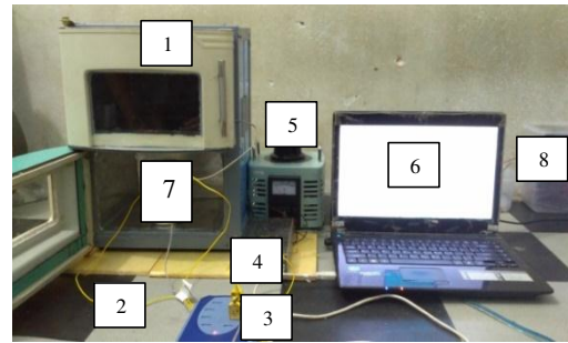
Gambar 3. Skema pengujian
