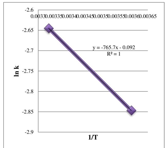
Gambar 4. Grafik hubungan 1/T dengan nilai ln k
