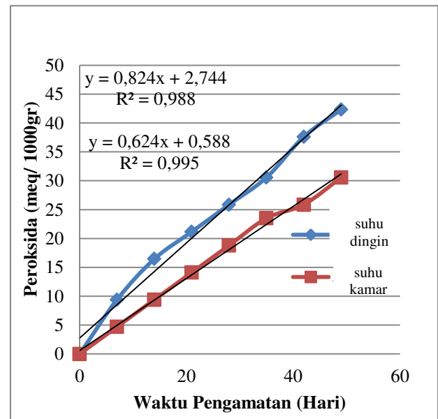
Gambar 2. Grafik hubungan antara waktu pengamatan (hari) dengan peroksida (meq/ 1000 g sampel) pada suhu kamar (27 °C) dan suhu dingin (5 °C)
