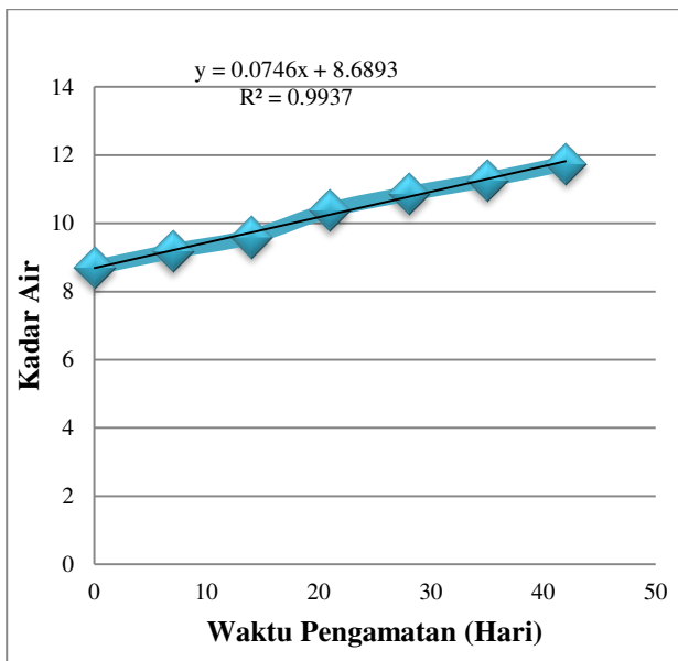
Gambar 1. Grafik hubungan antara waktu pengamatan (hari) dengan kadar air (%) pada suhu dingin (5 °C)
