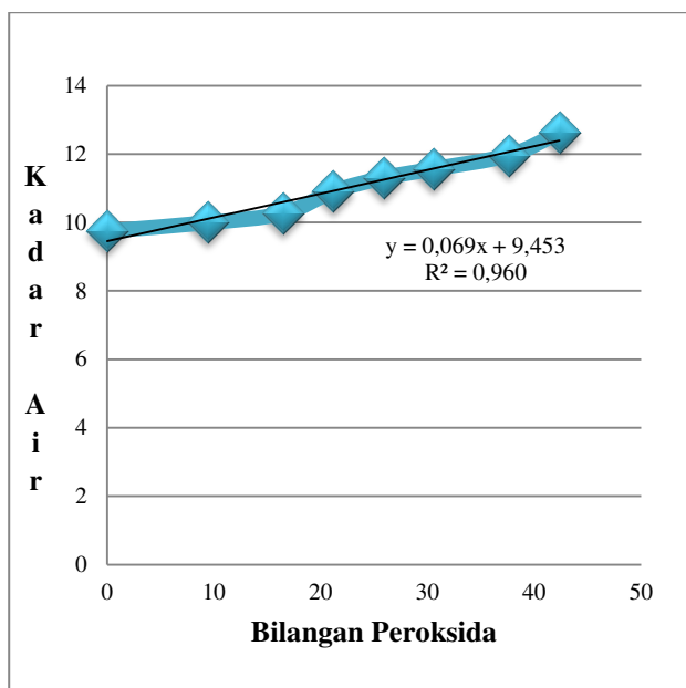
Gambar 5. Grafik hubungan antara bilangan peroksida dengan nilai kadar air pada suhu kamar (27 °C)
