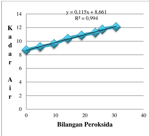
Gambar 6. Grafik hubungan antara bilangan peroksida dengan nilai kadar air pada suhu kamar (5 °C)
