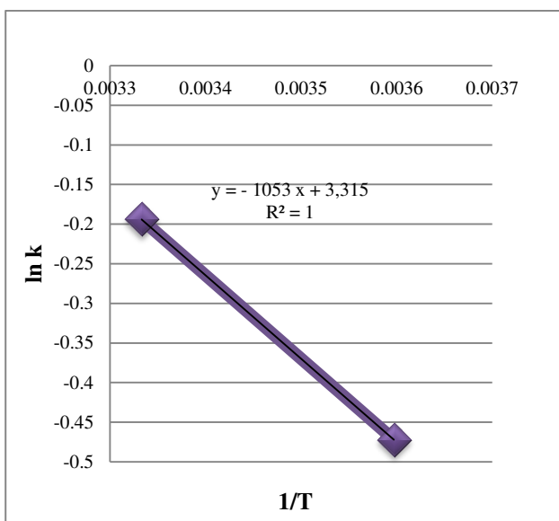
Gambar 3. Grafik hubungan 1/T dengan nilai ln k
