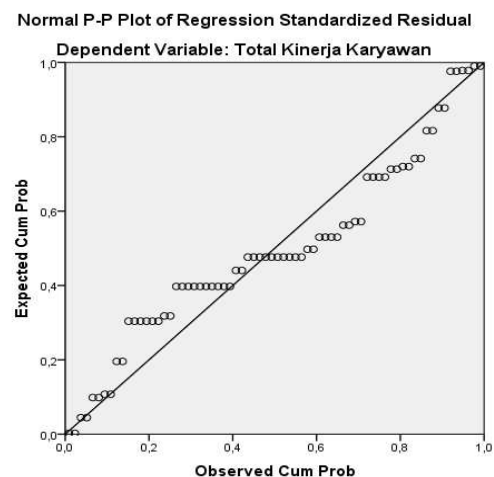
Gambar 3. Grafik Normal P-plot
