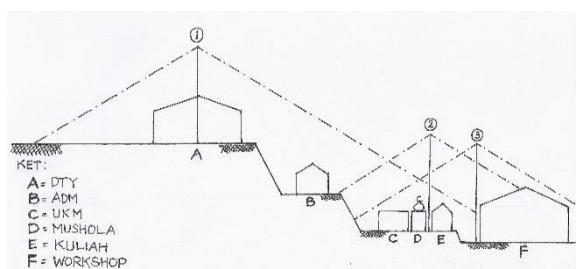
Gambar 7. Perancangan area cakupan proteksi petir pada gedung Politeknik Enjinerig Indorama
