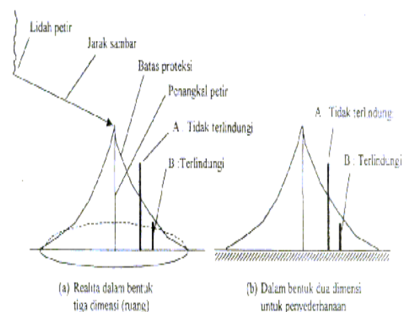
Gambar 2. Konsep ruang proteksi model elektromeometri (Hutauruk, 1991)
