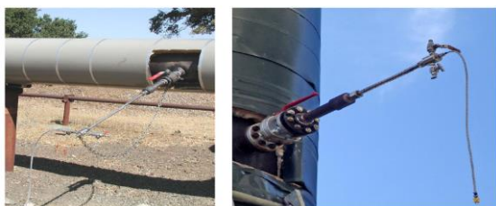
Gambar 4. Posisi sampling probe setelah dipasang dalam saluran pipa
