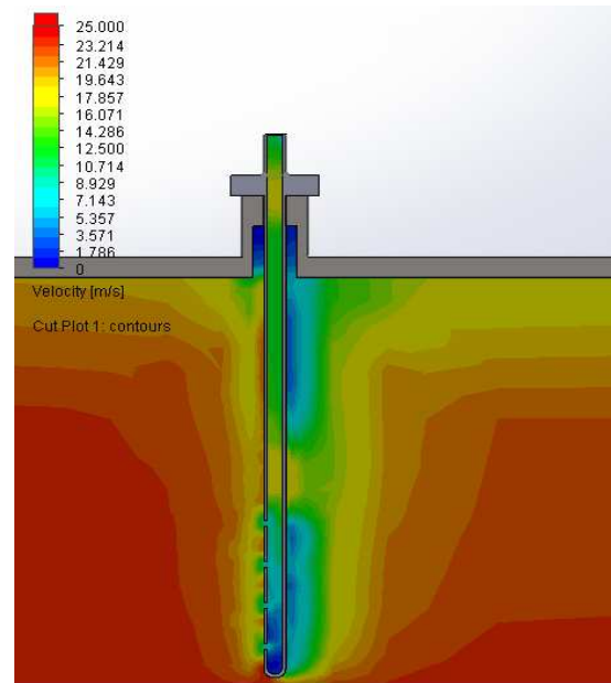
Gambar 12. Profil simulasi kecepatan fluida uap nozzle tip sampling probe diameter 0,125 inci
