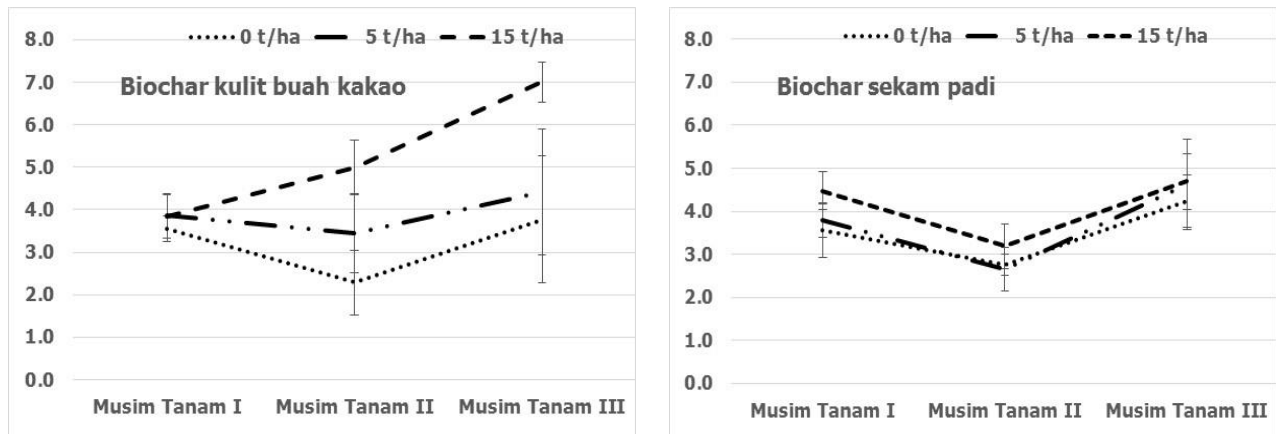
Gambar 1. Perkembangan hasil gabah kering panen setelah aplikasi biochar selama tiga musim tanam pada lahan sawah di KP Taman Bogo, Lampung Timur
