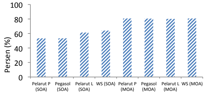
Gambar 2. Grafik solid content dari cat SOA dan MOA dengan menggunakan variabel pelarut
