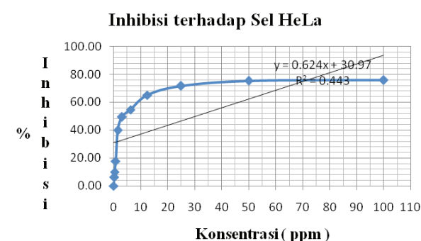
Gambar 1: Grafik hubungan konsentrasi terhadap % inhibisi
