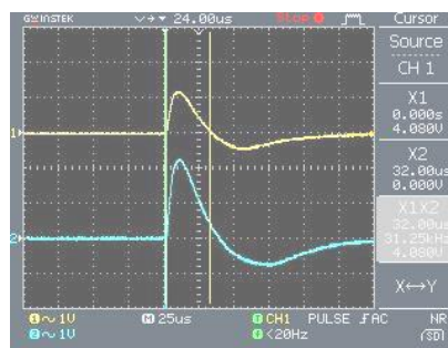
Gambar 5d. Lebar pulsa spot plasma sistem DUET pada permukaan katoda 2 ( \tau = 32 µs).
