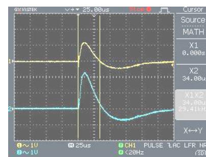
Gambar 6d. Lebar pulsa spot plasma sistem DUET pada permukaan katoda 2 ( \tau = 34 µs).
