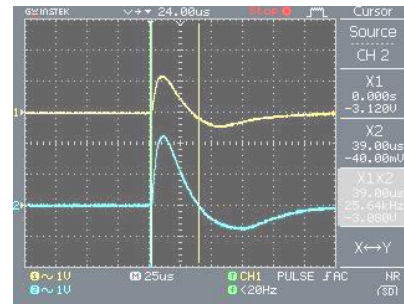
Gambar 5b. Lebar pulsa spot plasma sistem DUET pada permukaan katoda 1 ( \tau = 39 µs).
