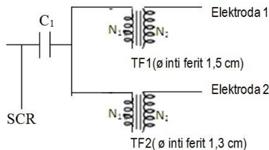
Gambar 3. Rangkaian sistem sumber daya ignitor (IDPS) sistem DUET.
