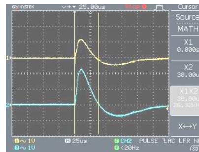
Gambar 6b. Lebar pulsa spot plasma sistem DUET pada permukaan katoda 1 ( \tau = 38 µs).
