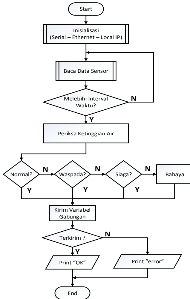
Gambar 5. Flowchart sistem yang diusulkan
