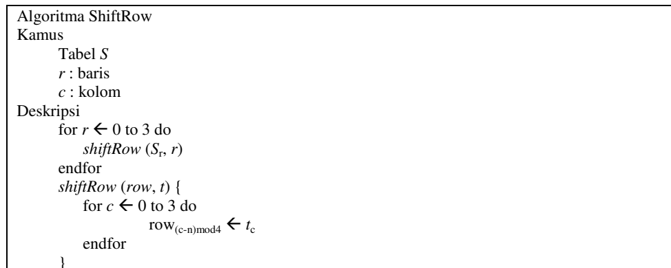
Gambar 5. Algoritma Transformasi Shift Row [5]
