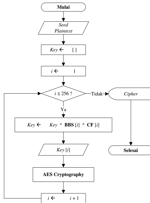
Gambar 9. Rancangan Modifikasi Kriptografi AES
