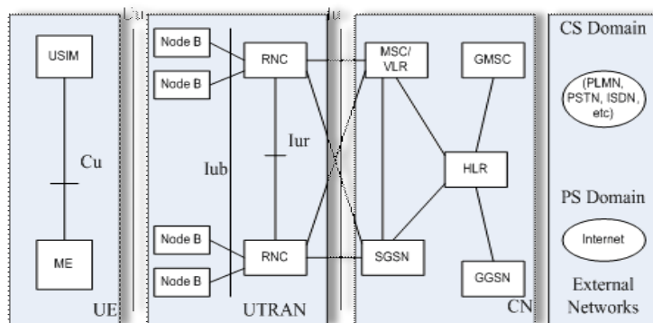
Gambar 1. Arsitektur Jaringan UMTS [1]
