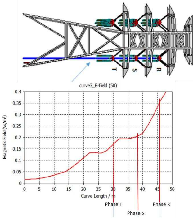
Gambar 12. Grafik Medan Magnet pada Phase R, S, dan T
