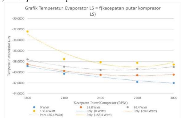
Gambar 4. Grafik Temperatur Evaporator LS = f (Kecepatan Putar Kompresor LS)
