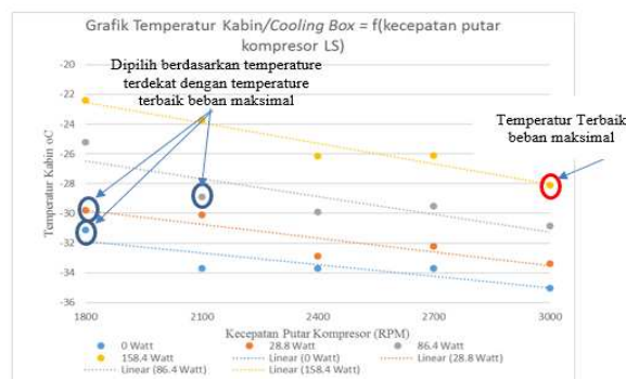
Gambar 12. Pemilihan Kecepatan Putar Kompresor Yang paling Sesuai Dengan Beban Pendinginan.
