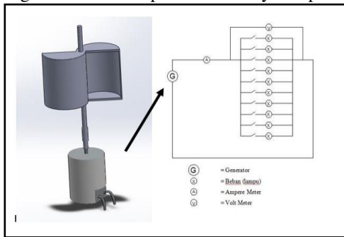
Gambar 5. Skema Rangkaian Pengukuran Daya
