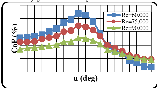
Gambar 11. Grafik nilai Coefficient of Power yang dihasilkan turbin Savonius sebagai fungsi sudut plat pengganggu
