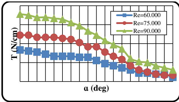
Gambar 10. Grafik nilai torsi statis yang dihasilkan turbin Savonius sebagai fungsi sudut plat pengganggu
