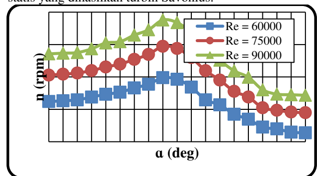
Gambar 9. Grafik nilai putaran yang dihasilkan turbin Savonius sebagai fungsi sudut plat pengganggu
