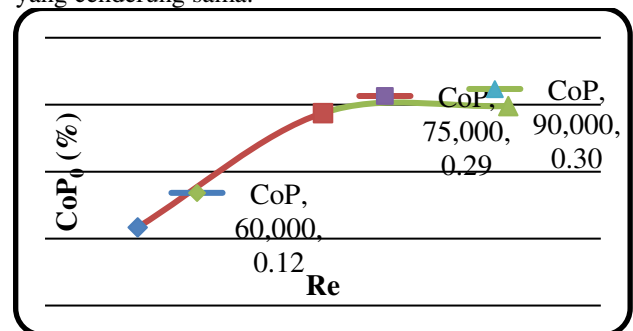
Gambar 8. Grafik nilai coefficient of power turbin Savonius tanpa plat pengganggu ( C_0P_0 ) sebagai fungsi Bilangan Reynolds (Re)
