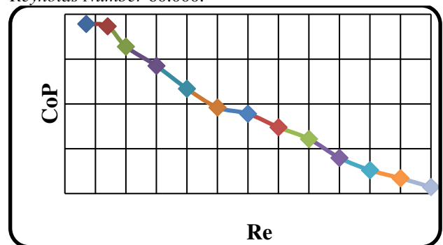
Gambar 15. Grafik nilai coefficient of power yang dihasilkan turbin Savonius sebagai fungsi Reynolds Number pada sudut plat pengganggu 40°
