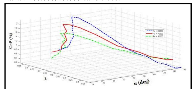
Gambar 16. Grafik nilai coefficient of power yang dihasilkan turbin Savonius sebagai fungsi tip speed ratio
