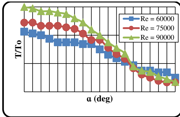
Gambar 13. Grafik nilai peningkatan torsi statis yang dihasilkan turbin Savonius sebagai fungsi sudut plat pengganggu
