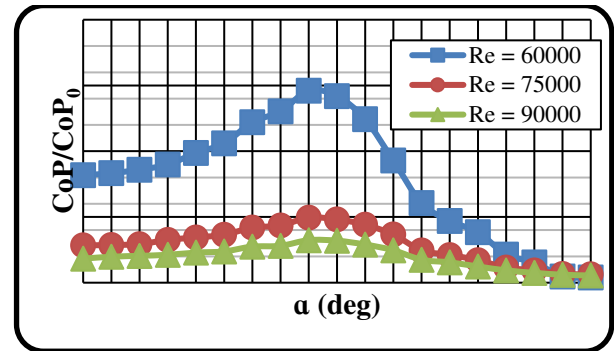
Gambar 14. Grafik peningkatan nilai Coefficient of Power yang dihasilkan turbin Savonius sebagai fungsi sudut plat pengganggu
