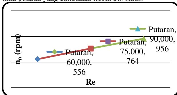
Gambar 6. Grafik putaran turbin Savonius tanpa plat pengganggu ( n_0 ) sebagai fungsi Bilangan Reynolds (Re)
