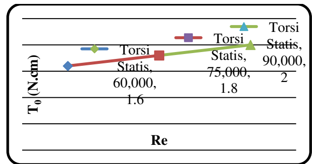
Gambar 7. Grafik torsi statis turbin Savonius tanpa plat pengganggu ( T_0 ) sebagai fungsi Bilangan Reynolds (Re)
