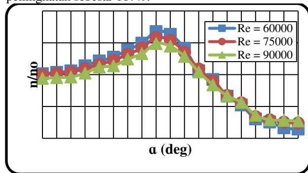
Gambar 12. Grafik peningkatan nilai putaran yang dihasilkan turbin Savonius sebagai fungsi sudut plat pengganggu
