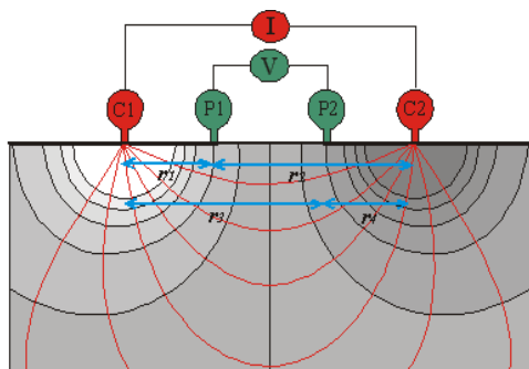
Gambar 1 Konfigurasi elektroda Schlumberger
