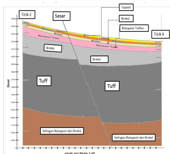
Gambar 3. Penampang bawah permukaan lintasan II (4-2)
