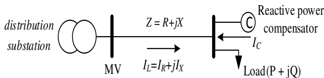
Gambar 2 Pemasangan kapasitor secara paralel
