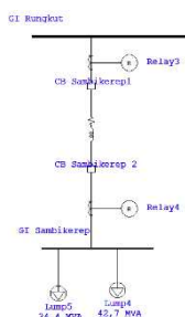
Gambar 3.4 Single line diagram Gardu Induk Rungkut ke Gardu Induk Sambikerep
