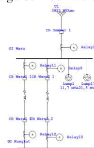
Gambar 3.1 Single line diagram Gardu Induk Waru ke Gardu Induk Runkut
