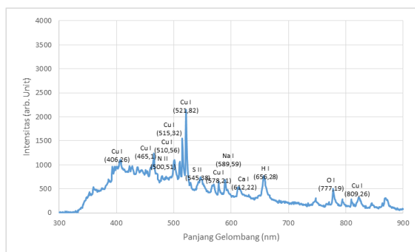
Gambar 3. Grafik spektrum plat tembaga (10 Hz, 75%, 1 atm)
