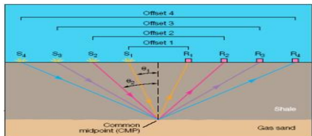
Gambar 2 Hubungan antara offset dengan sudut datang ( \theta ) dan sinyal datang yang terekam dalam titik reflektor yang sama (Chiburis et al., 1993) [5].
