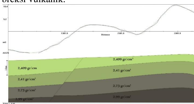
Gambar 6 Pemodelan 2D Data Gravitasi pada Sayatan A
