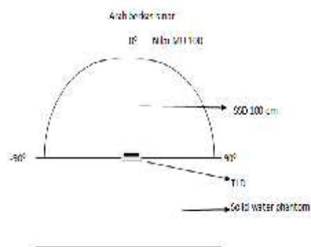
Gambar 2. Set up pengukuran koreksi sudut datang
