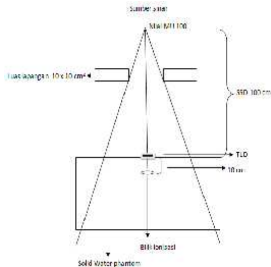
Gambar 1. Set up pengukuran kalibrasi
