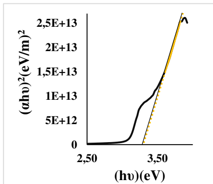
Gambar 5 Plot (\alpha h\nu)^2 vs h\nu lapisan tipis bilayer ZnO/TiO 2
