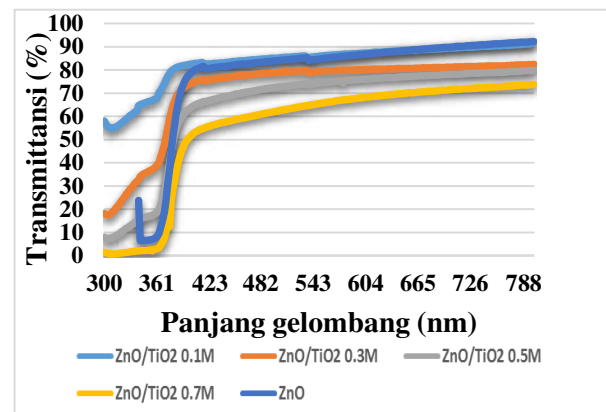
Gambar 3 Transmitansi UV-Vis lapisan tipis bilayer ZnO/TiO 2 dengan variasi konsentrasi ZnO
