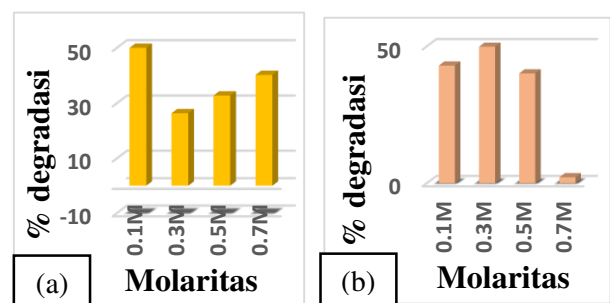
Gambar 8 Tingkat degradasi lapisan bilayer ZnO/TiO 2 (a) zat warna methyl orange dan (b) pewarna batik
