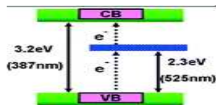
Gambar 4 Peristiwa trapping electron
