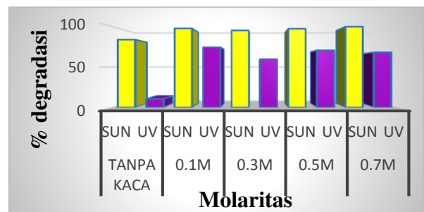
Gambar 7 Tingkat kecepatan fotodegradasi lapisan bilayer ZnO/TiO 2 terhadap zat warna methylene blue
