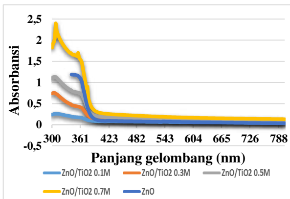
Gambar 2 Spektrum absorbansi UV-Vis lapisan tipis bilayer ZnO/TiO 2 dengan variasi konsentrasi ZnO
