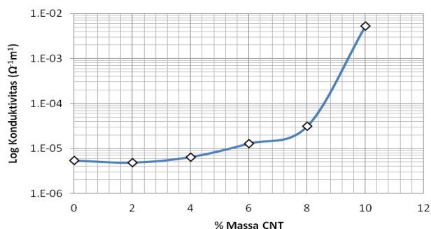
Gambar 4.1 Grafik hubungan komposisi % massa CNT dalam komposit CNT-PVDF terhadap nilai konduktivitas
