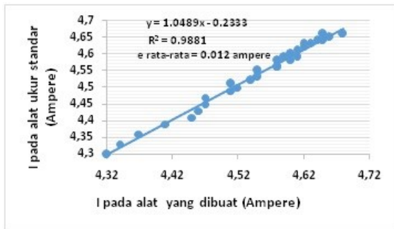
Gambar 5. Grafik kalibrasi sensor arus
