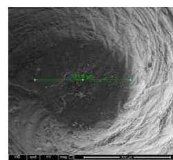
Gambar 13. Permukaan elektrode kuningan sesudah diberi tegangan pra-peluahan
