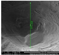
Gambar 17. Permukaan elektrode baja sesudah diberi tegangan pra-peluahan
