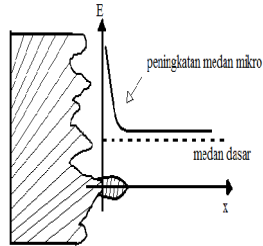
Gambar 5. Peningkatan medan karena kekasaran elektroda
