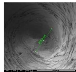
Gambar 16. Permukaan elektrode baja sebelum diberi tegangan pra-peluahan
