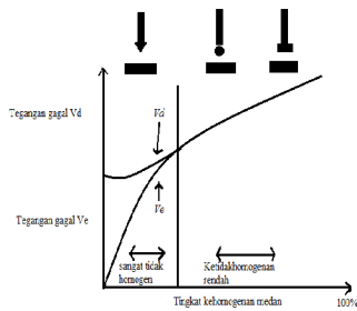
Gambar 2. Tegangan gagal dan tegangan mula pra-kegagalan tergantung pada tingkat kehomogenan
