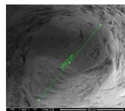
Gambar 15. Permukaan elektrode aluminium sesudah diberi tegangan pra-peluahan
