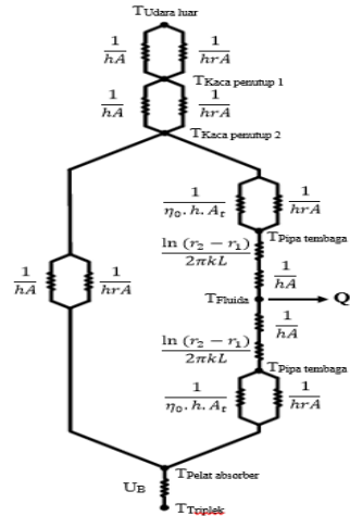
Gambar 3 Skema tahanan termal dua kaca penutup
