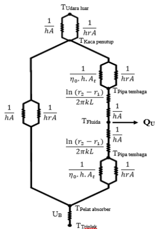
Gambar 2 Skema tahanan termal satu kaca penutup
