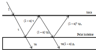
Gambar 1 Penyerapan radiasi oleh pelat penyerap[1]
