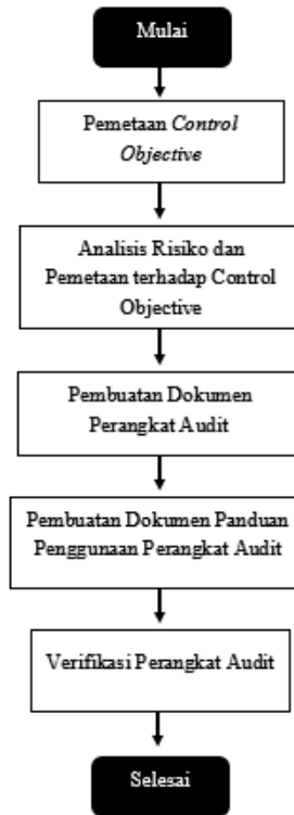
Gambar 2. Metodologi Penelitian
