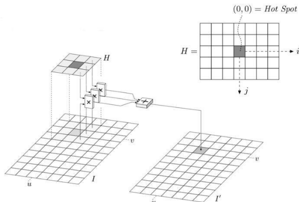
Gambar 4. Visualisasi konvolusi citra
