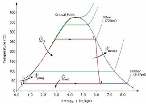
Gambar 3 Grafik T-s Siklus Rankine
