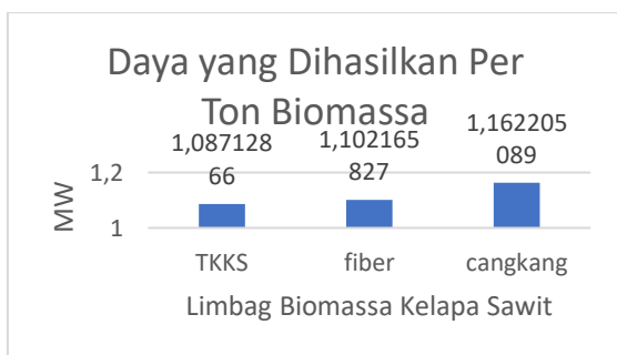
Gambar 7 Grafik Daya yang Dibangkitkan
