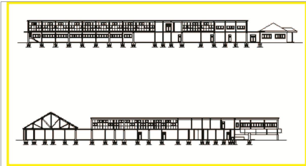
Gambar 18: Potongan bangunan Rumah Sakit Hewan di Kota Pontianak
