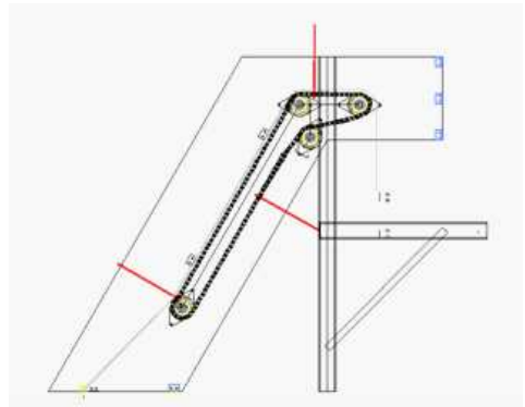
Gambar 2. Kontruksi Konveyor 1
