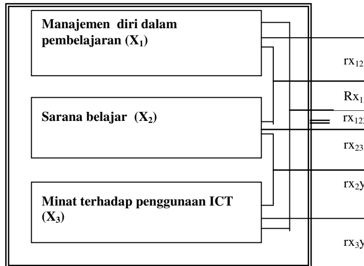
Gambar 1. Hubungan Antarvariabel
