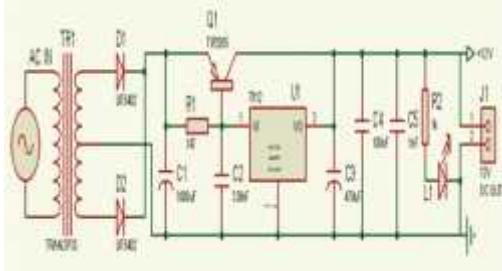
Gambar 3.2 Skema Rangkaian Catu Daya
