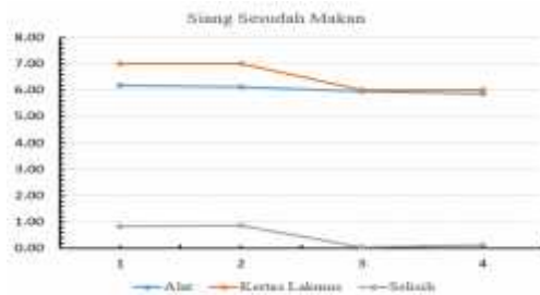
Gambar 4.8 Grafik siang sesudah makan
