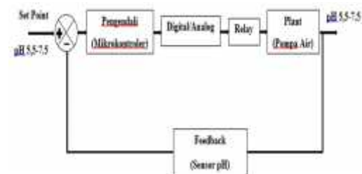
Gambar 3.1 Blok Diagram Sistem Perencanaan
