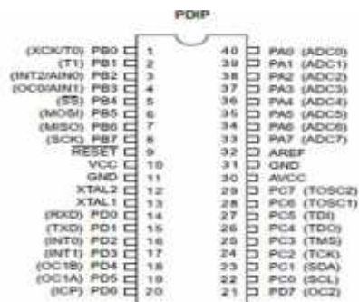
Gambar 2.3 Konfigurasi Fungsi Kaki Pin ATmega16
