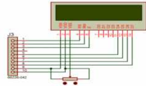
Gambar 3.4 Skema Rangkaian LCD monitor 16x2 karakter.
