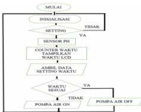
Gambar 3.6 Diagram Alir Program Utama
