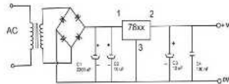
Gambar 1.1 Catu Daya Teregulasi Tegangan Positif
