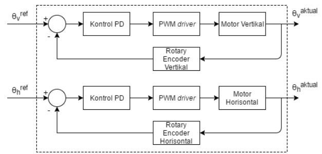
Gambar 6. Diagram Pengarahan Senjata ke Target
