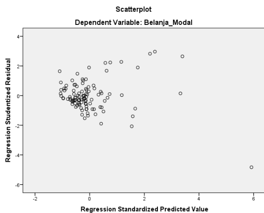
Gambar 1. Diagram Heteroskedastisitas
