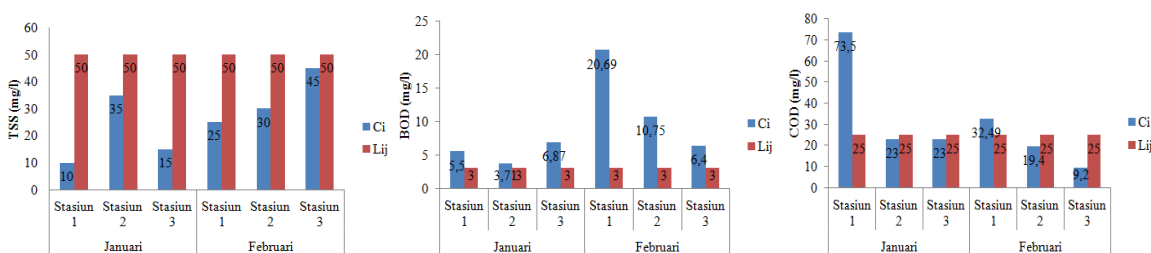
Gambar 3. Histogram Perbandingan Ci dan Lij parameter TSS, BOD, dan COD
