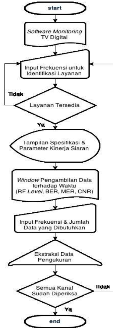
Gambar 3. Flowchart pengukuran lapangan kinerja siaran TV digital
