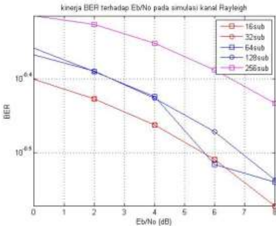
Gambar 10. Kinerja BER terhadap Eb/No pada kanal Rayleigh di subcarrier yang berbeda
