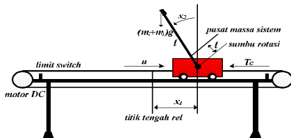
Gambar 1. Diagram fisik sistem pendulum kereta
