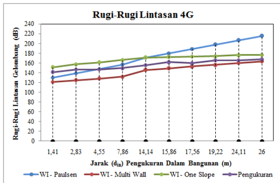
Gambar 14. Pathloss Sektor 3 Sistem 4G
