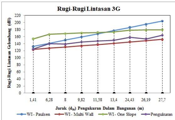
Gambar 15. Pathloss Sektor 1 Sistem 3G
