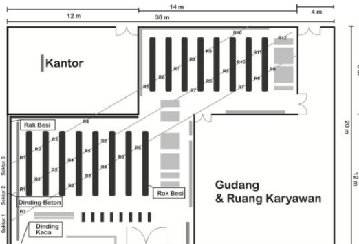
Gambar 5. Denah Bangunan Mitra mart
