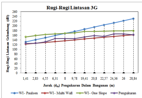
Gambar 16. Pathloss Sektor 2 Sistem 3G
