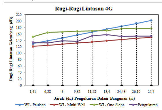
Gambar 12. Pathloss Sektor 1 Sistem 4G
