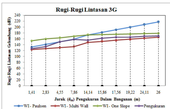
Gambar 17. Pathloss Sektor 3 Sistem 3G
