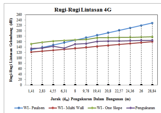
Gambar 13. Pathloss Sektor 2 Sistem 4G
