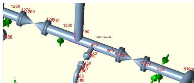
Gambar 13. Tegangan operasional .
