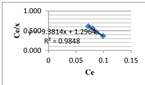
Gambar 4. Grafik Linearisasi Isoterm Langmuir
