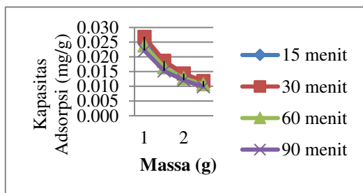
Gambar 3. Perbandingan Kapasitas Adsorpsi Variasi Massa Adsorben dan Waktu Kontak Terhadap Penurunan Fe
