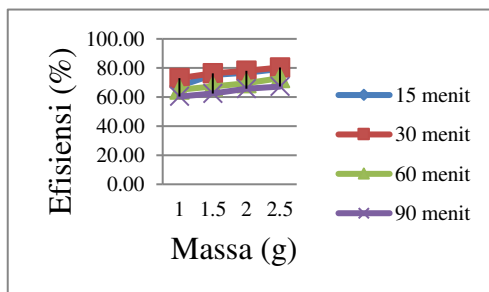
Gambar 1. Grafik Hubungan Antara Massa Adsorben Terhadap Efisiensi Penurunan Fe
