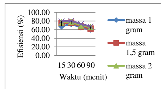
Gambar 2. Grafik Hubungan Antara Waktu Kontak Terhadap Efisiensi Penurunan Fe
