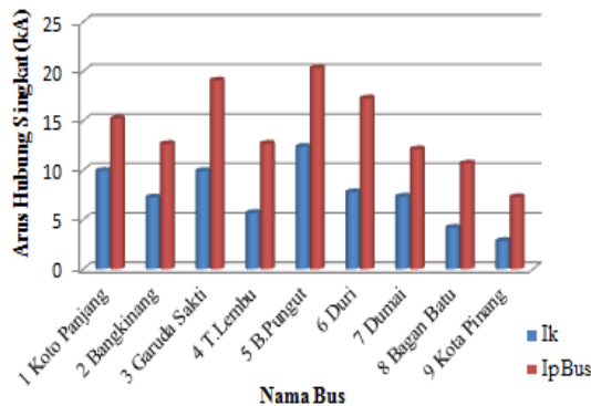
Gambar 4.1 arus hubung singkat pada masing-masing Bus sistem wilayah Riau kondisi 1
