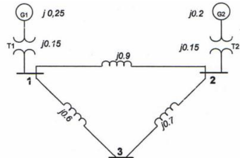
Gambar 2.5 Diagram impedansi sebuah sistem tenaga listrik sederhana
