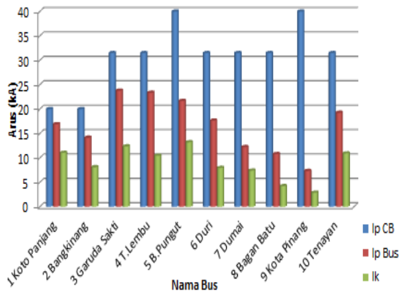
Gambar 4.4 Perbandingan besar arus pada masing-masing bus kondisi 2
