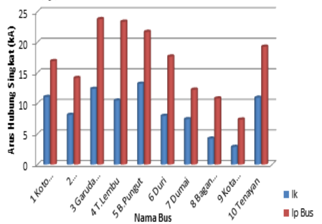
Gambar 4.3 Arus hubung singkat pada masing-masing Bus sistem wilayah Riau kondisi II
