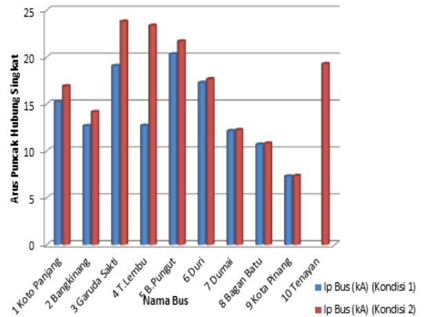
Gambar 4.6 Perbandingan arus puncak hubung singkat pada bus subsistem Riau kondisi I dan kondisi II
