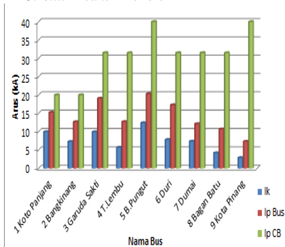
Gambar 4.2 Perbandingan besar arus pada masing-masing bus kondisi 1
