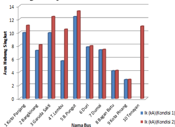
Gambar 4.5 Perbandingan arus hubung singkat pada bus subsistem Riau kondisi I dan kondisi II
