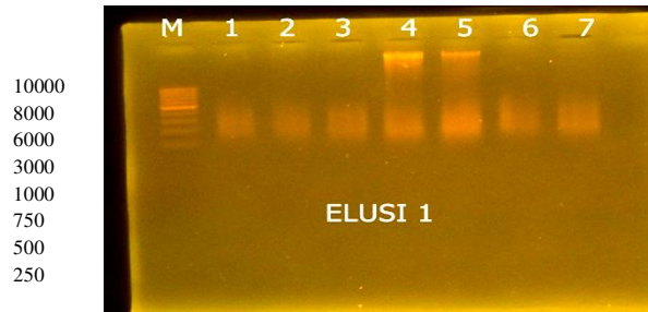
Gambar 2. Hasil Elektroforesis DNA Total isolat Bakteri dengan konsentrasi agarose 1,2% , marker DNA 1kb ladder.
