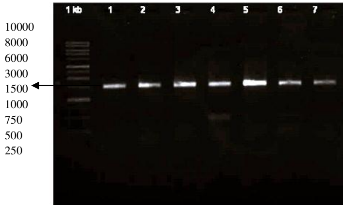
Gambar 3. Hasil Elektroforesis Produk PCR
