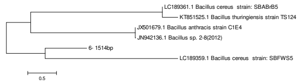
Gambar 9. Pohon filogenetik isolat D6
