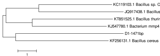
Gambar 4. Pohon filogenetik isolat D1
