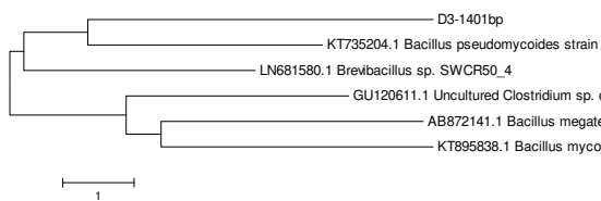
Gambar 6. Pohon filogenetik isolat D3
