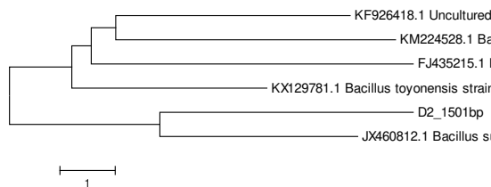
Gambar 5. Pohon filogenetik isolat D2
