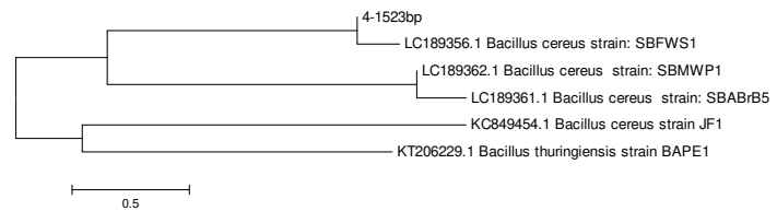
Gambar 7. Pohon filogenetik isolat D4
