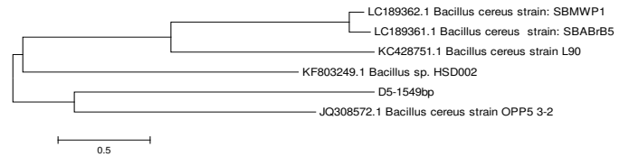
Gambar 8. Pohon filogenetik isolat D5
