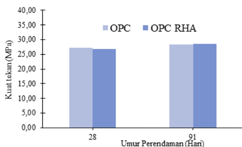
Gambar 3. Grafik hasil kuat tekan mortar rendaman air biasa
