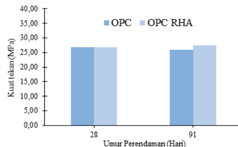
Gambar 4. Hasil kuat tekan mortar rendaman air gambut
