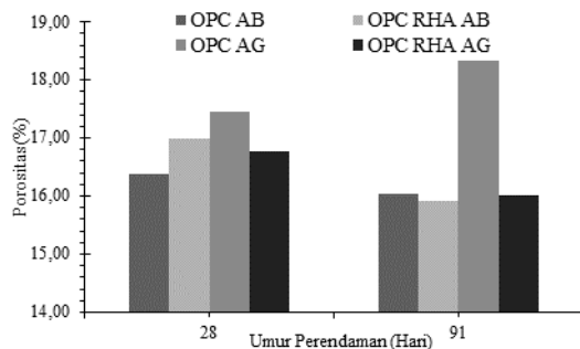
Gambar 5. Grafik hasil pengujian porositas dalam rendaman air biasa maupun air gambut
