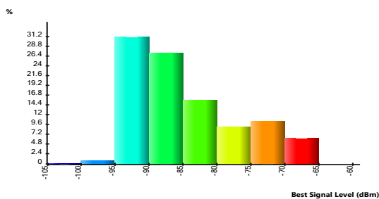
Gambar 8. Histogram nilai Cakupan sinyal skenario FFR
