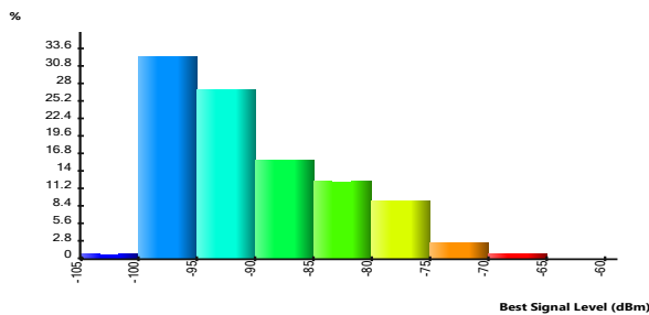
Gambar 7. Histogram nilai Cakupan sinyal skenario FR1
