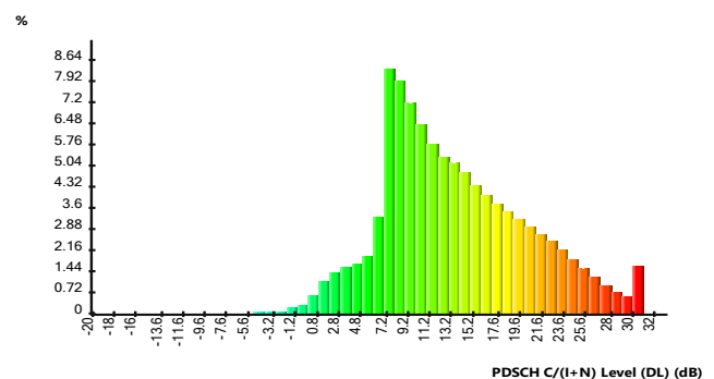
Gambar 9. Histogram nilai CINR skenario FR1
