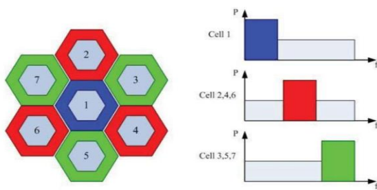
Gambar 3. Perencanaan frekuensi dan alokasi daya pada skema SFR
