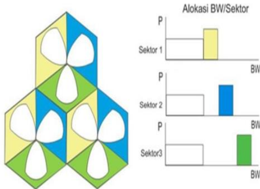
Gambar 5. Alokasi Power dan Frekuensi pada FFR
