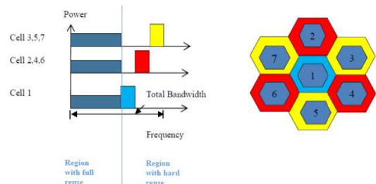
Gambar 2. Perencanaan frekuensi dan alokasi daya pada skema PFR
