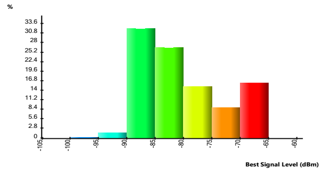
Gambar 9. Histogram nilai Cakupan sinyal skenario SFR
