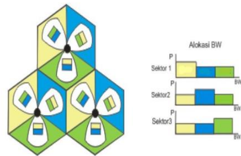
Gambar 6. Alokasi Power dan Frekuensi pada SFR
