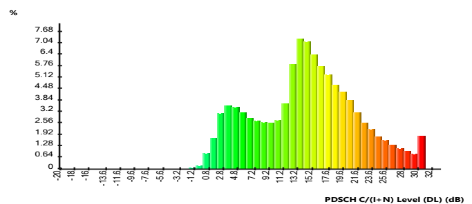
Gambar 11. Histogram nilai CINR skenario FFR
