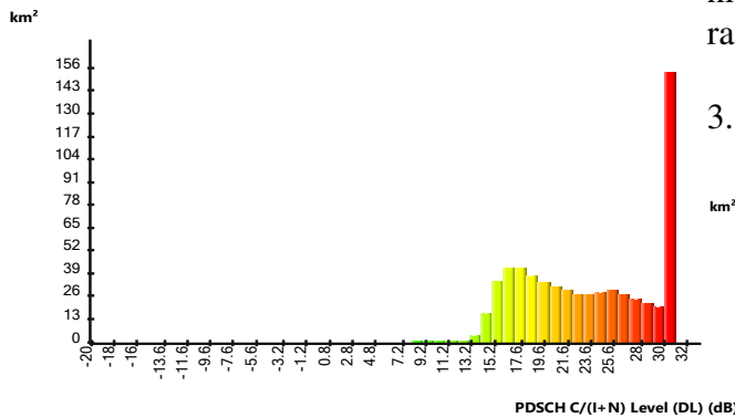
Gambar 12. Histogram nilai CINR skenario SFR
